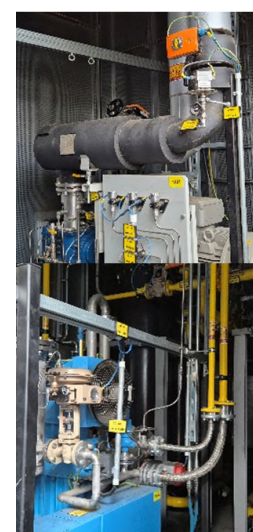
La station GRDF de contrôle, d'odorisation, de comptage et d'injection du gaz dans le réseau de distribution 4 bar.
